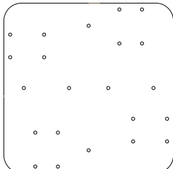
層板正面 (沉孔朝下)
